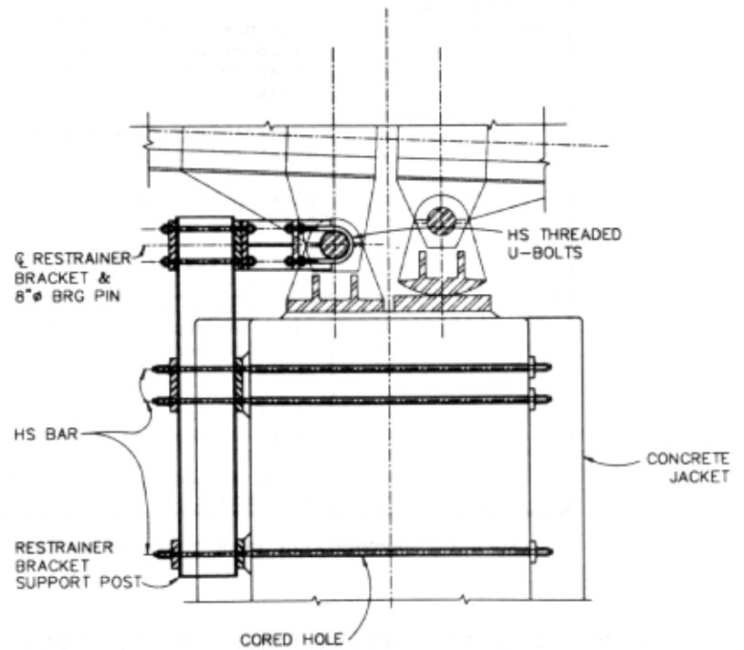
LONGITUDINAL RESTRAINER BRACKET
